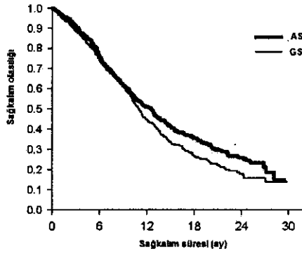
Adenokarsinoma
