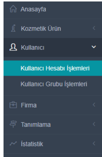
Şekil 12. Kullanıcı İşlemler
